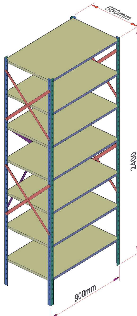
PERSPECTIVA - Isométrica SEM ESCALA
