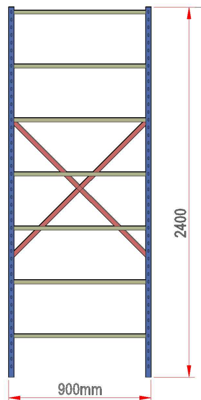
FRONTAL - Vistas ESCALA 1/25
