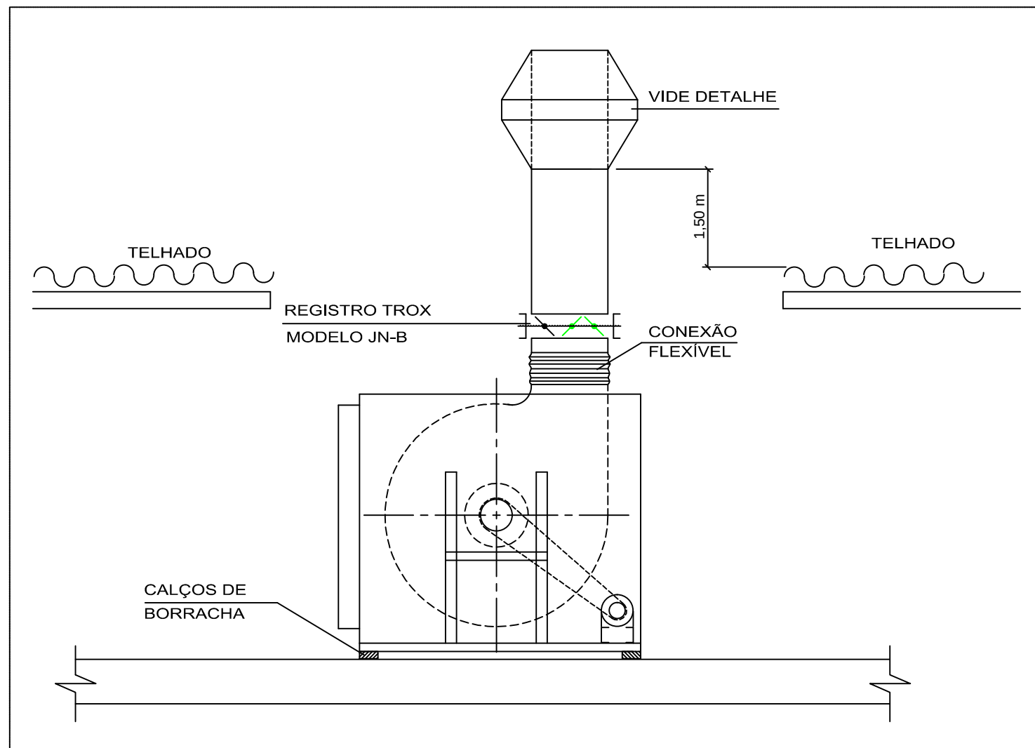
DETALHE TÍPICO DA POSIÇÃO DA CAIXA DE EXAUSTÃO SEM _____ ESCALA
